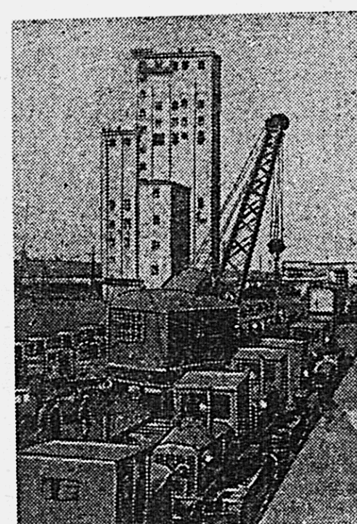
Алтайский край. В городе Рубцовске за годы Отечественной войны выросло крупное предприятие — Алтайский тракторный завод, который уже дал стране тысячи тракторов. На снимке: погрузка тракторов на платформу. (Фото О. Вейсмана. (Фотокорреспондент ТАСС).
