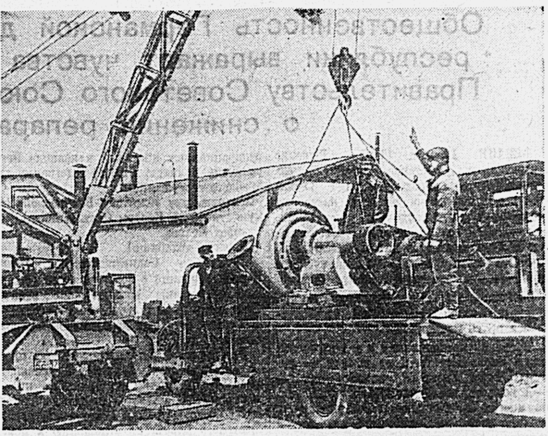
Хабаровский механический завод «Главострыбтары» освоил серийное производство рыбоконсервов. На Камчатку и Сахалин уже отправлены десятки новых машин. На снимке: погрузка на автомашину спаренной рыбоконсервной установки для отправки в Нижне-Амурскую область. Фото А. Каминкова.
