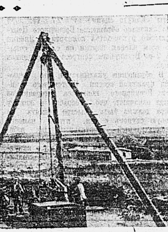
Украинская ССР. На месте строительства будущей Каховской гидроэлектростанции приняты первые разведочные скважины в районе будущей Каховской гидроэлектростанции. На снимке: бурение разведочных скважин в районе будущей Каховской гидроэлектростанции. Фото Я. Давидова. (Фотохроника ТАСС).
