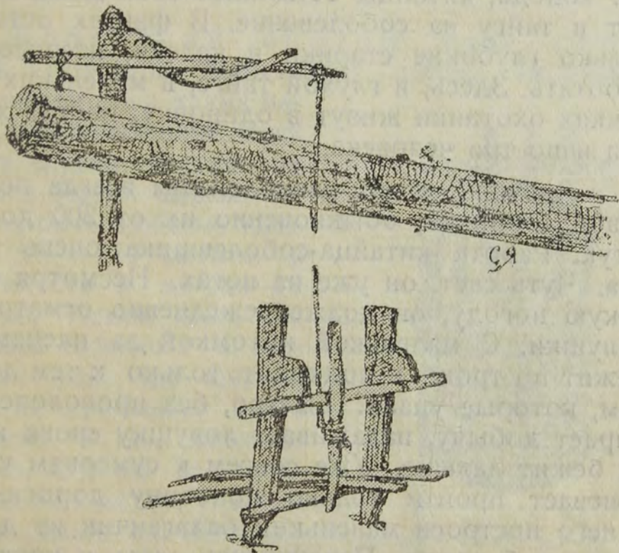
Механизм китайской ловушки на соболя, приводящий ее в действие,
