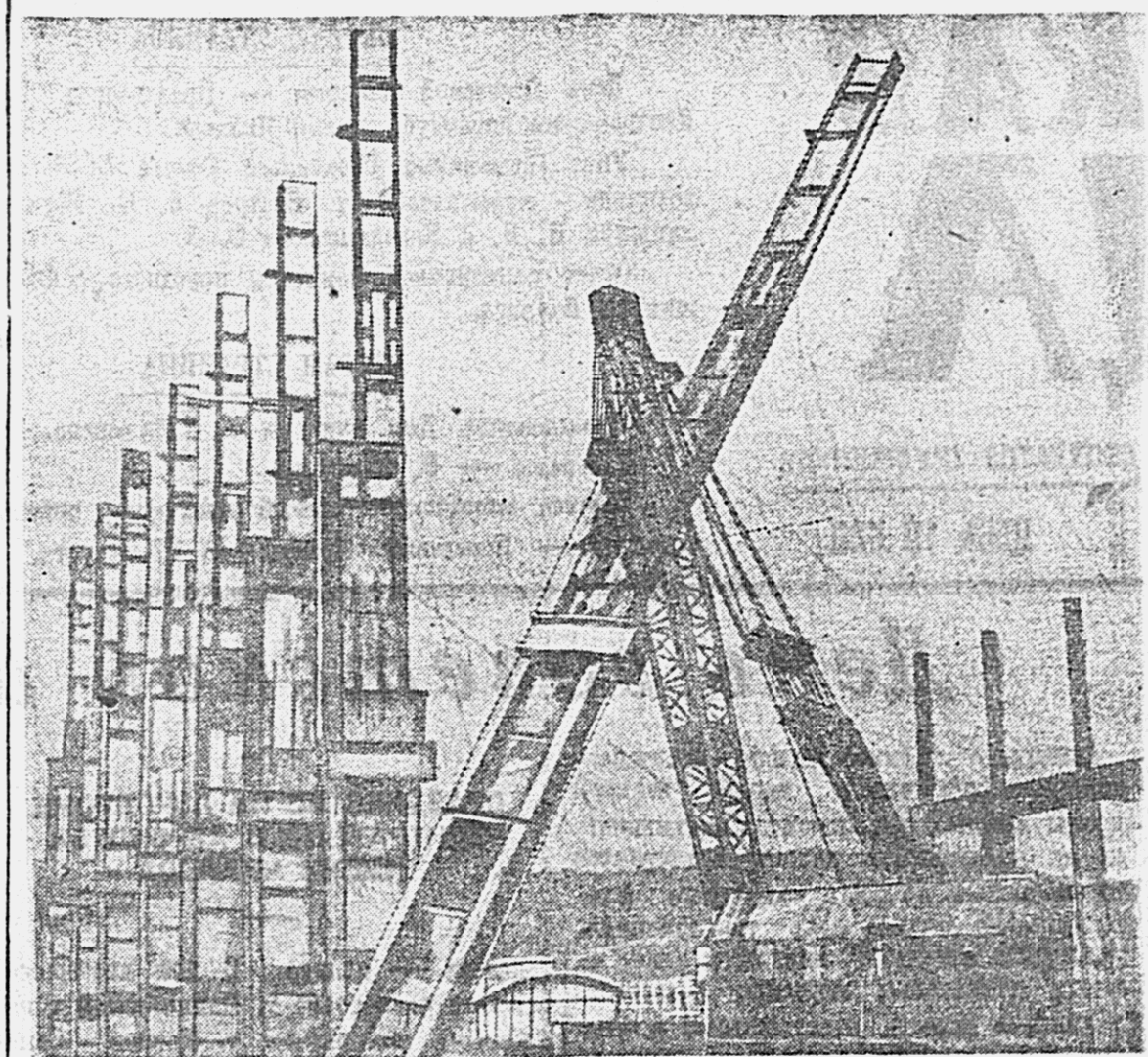
Амурстальстрой. На снимке: подъем и установка колонн на мартене. Фото В. Григорьева.
